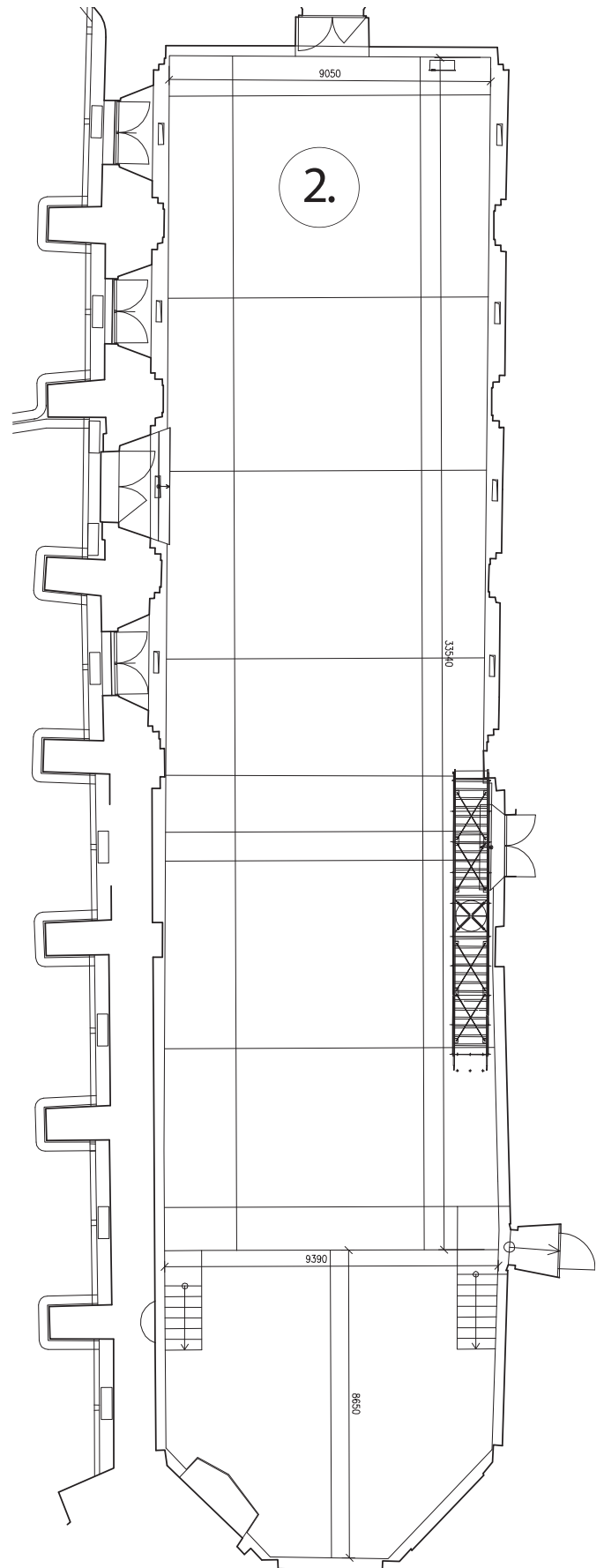
2. Půdorys hlavní lodi kostela
